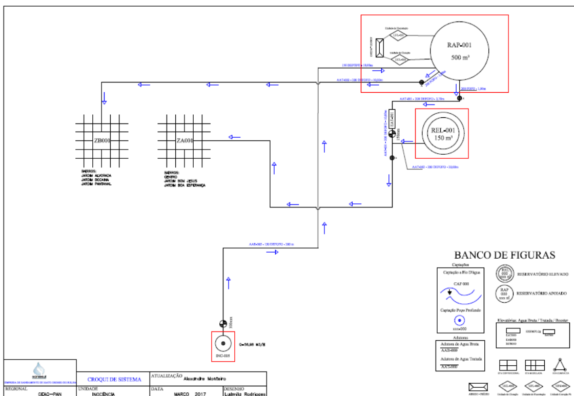
Fluxograma do processo do Sistema de Abastecimento de Água de Aquidauana.
