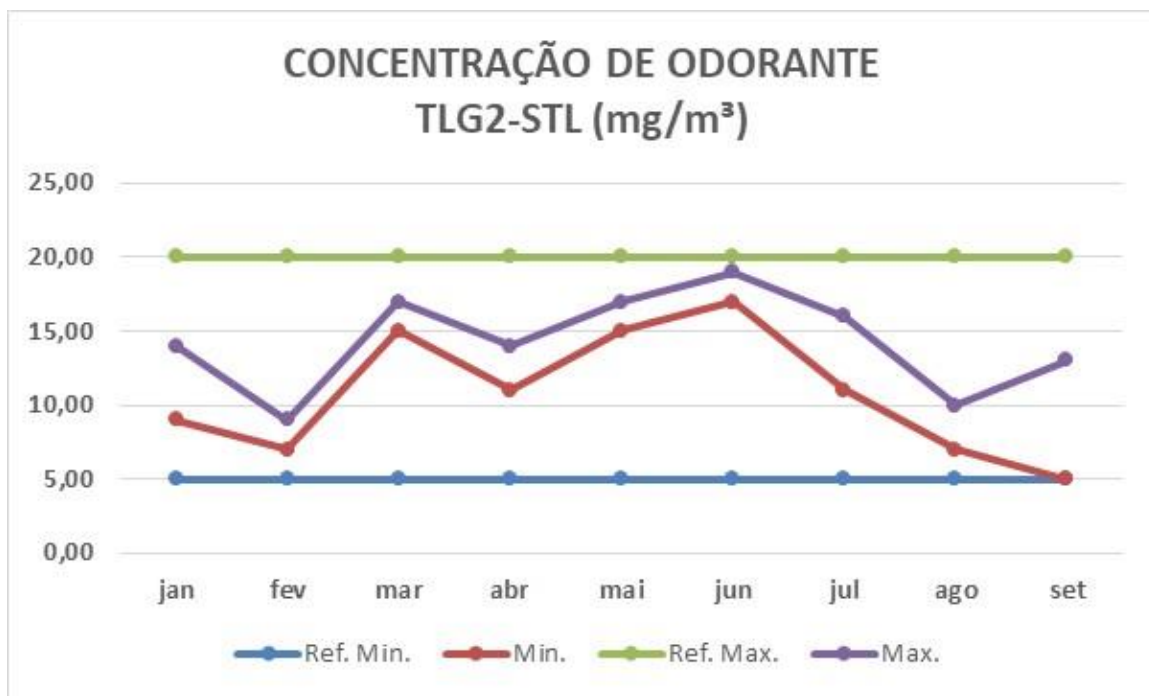
Gráfico 34: Concentração de Odorante no Gás (COG) – Estação STL (Siderúrgica Sitrrel de Três Lagoas)
