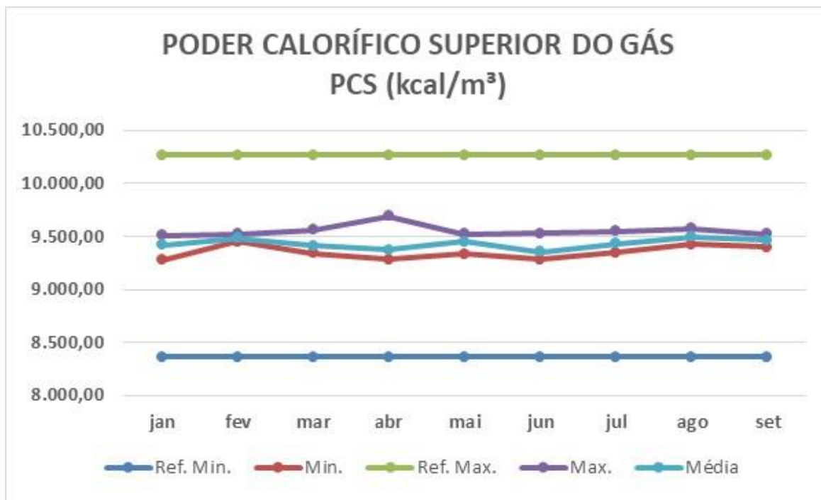
Gráfico 24: Poder Calorífico Superior (PCS) do gás canalizado
