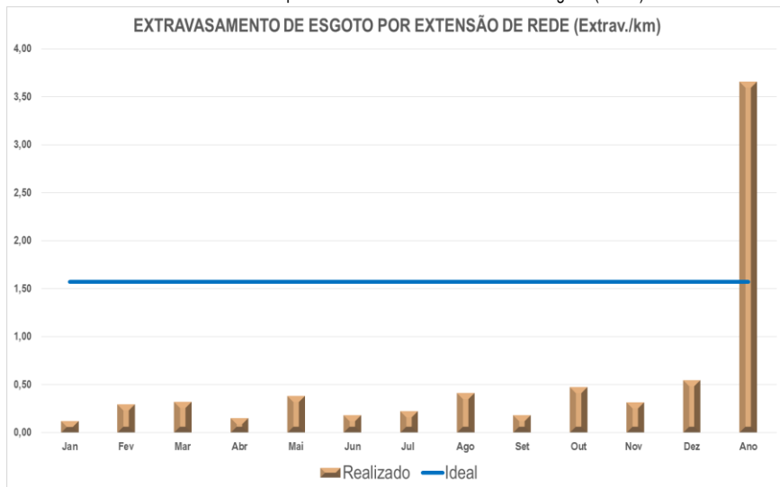
Gráfico 13 – Desempenho mensal de Extravasamento de esgoto (IN082).
