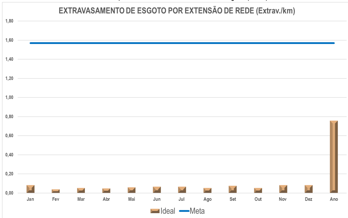
Gráfico 13 – Desempenho mensal de Extravasamento de esgoto (IN082).
